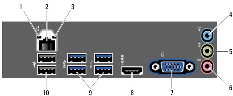
Рисунок 2. Вид задней панели
